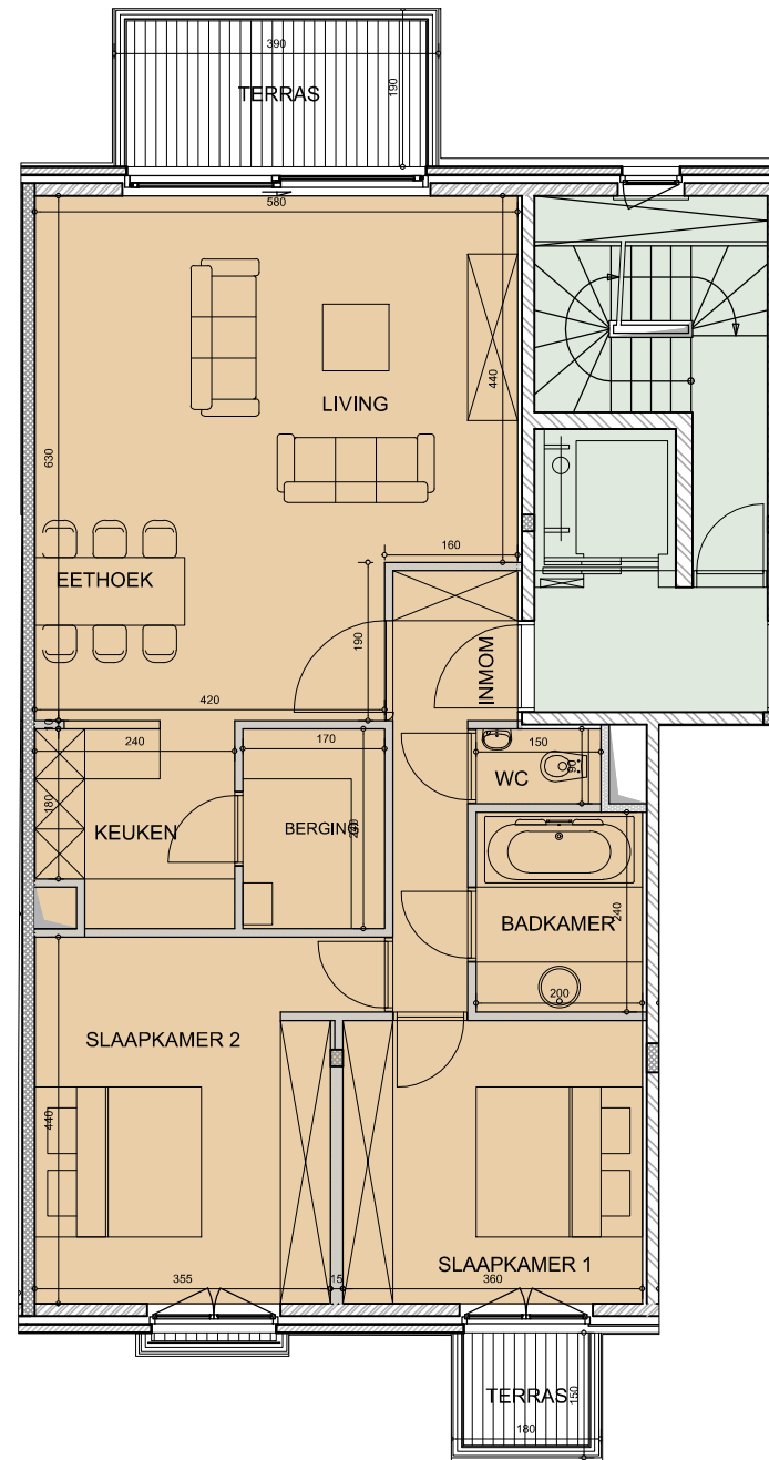
Eerste verdieping appartement 4/4 0102, schaal 1/100
