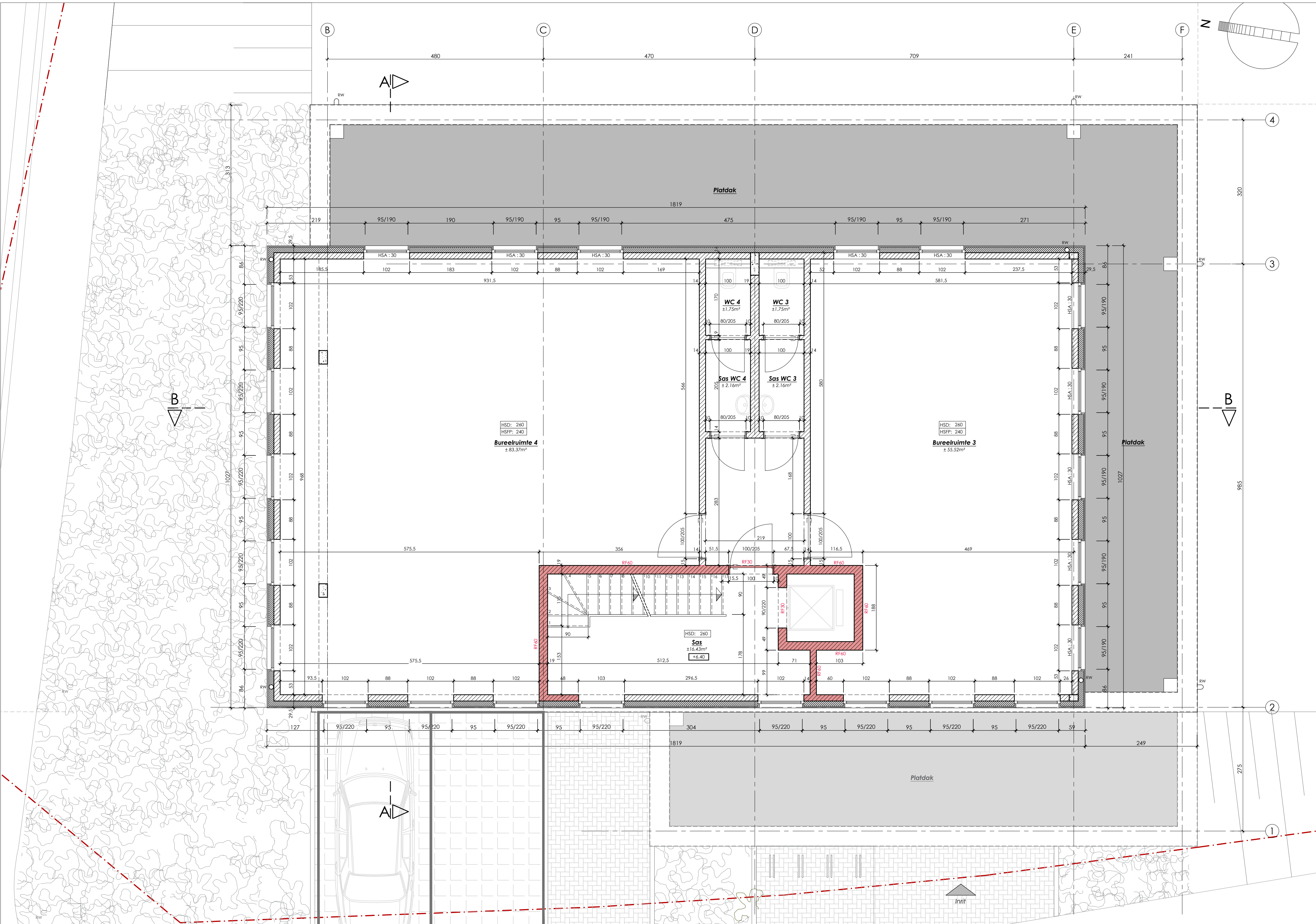
Tweede verdieping - 1/50
