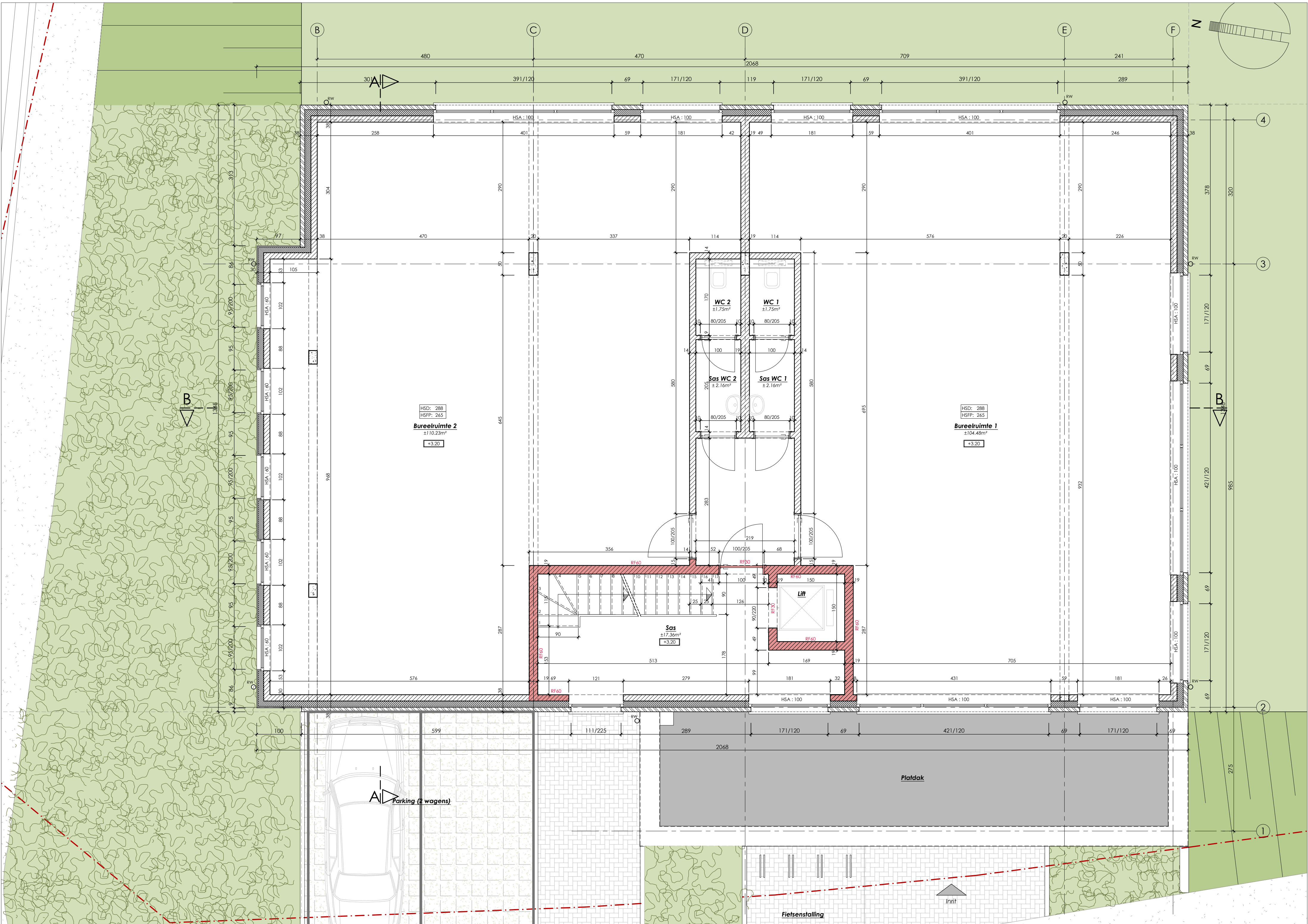
Eerste verdieping - 1/50
