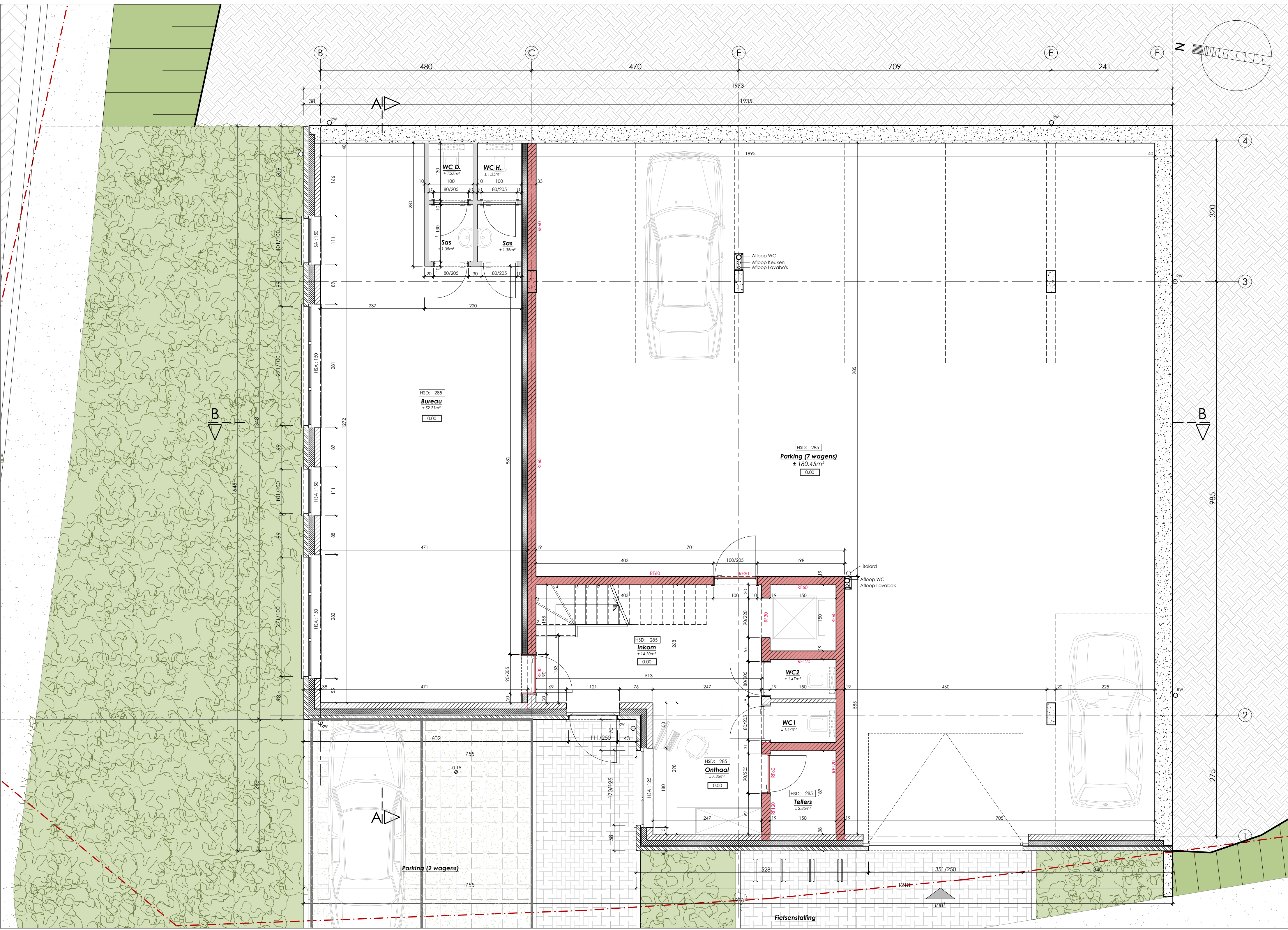
Gelijkvloerse verdieping - Garage niveau - 1/50
