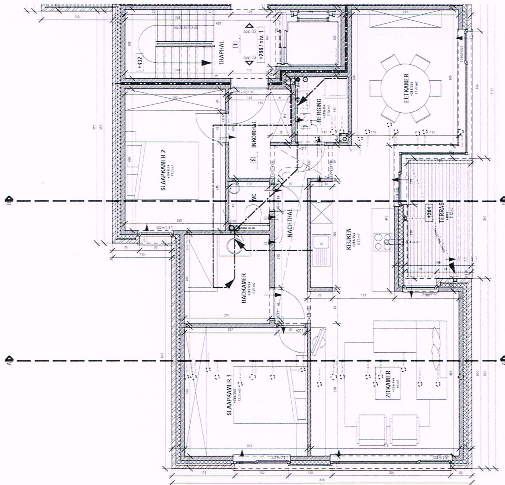
1e verdieping - appartement 3 schaal 1/100
