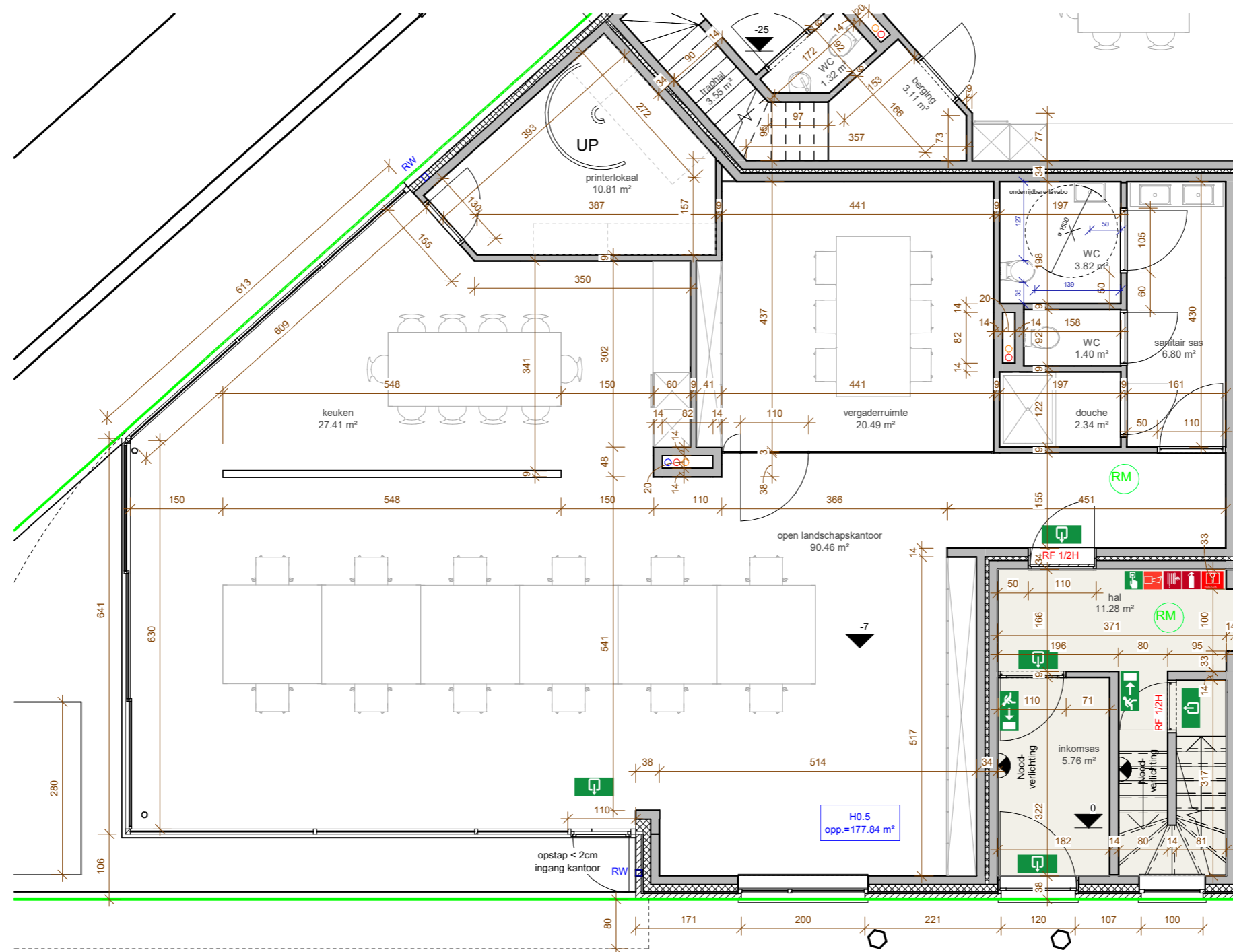
1 gelijkvloers 1 : 75
