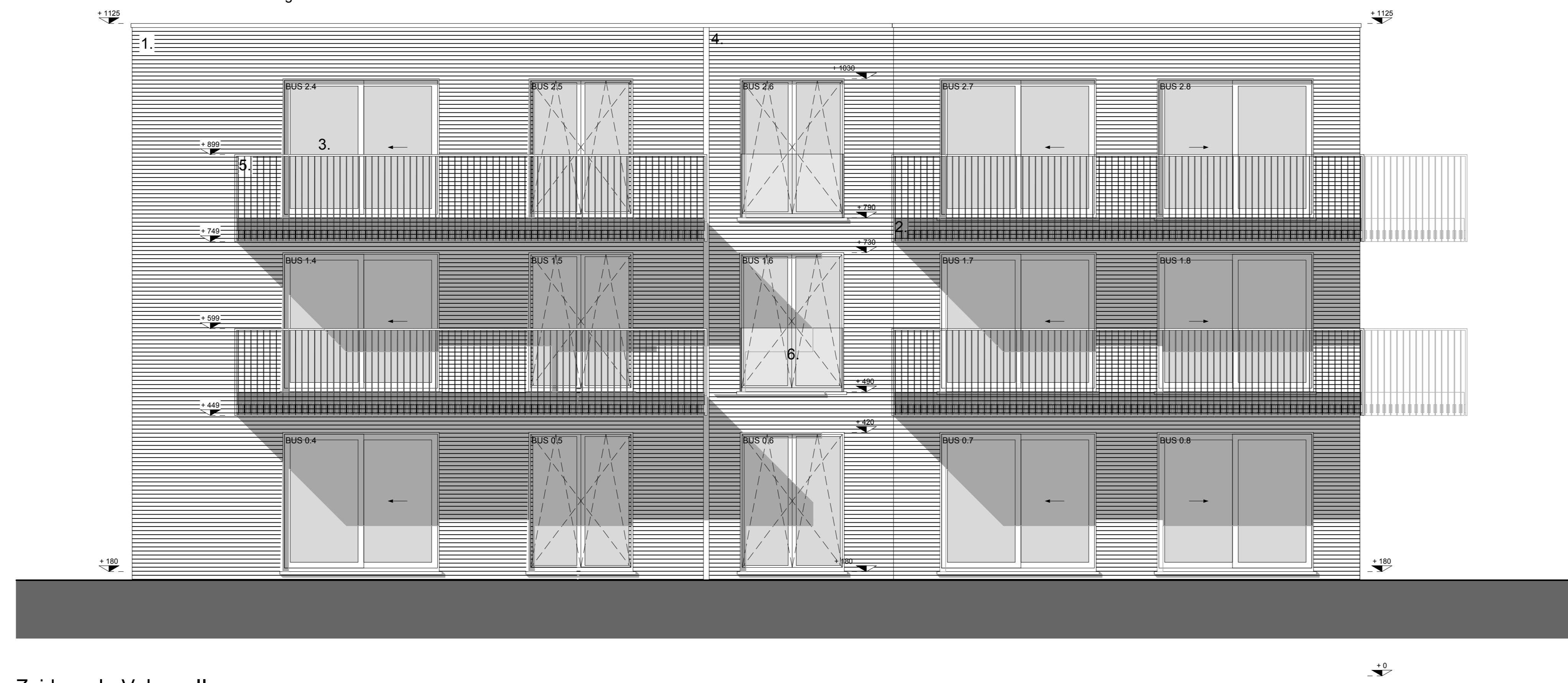
Zuidgevel - Volume II 0 0.5 2.5m
