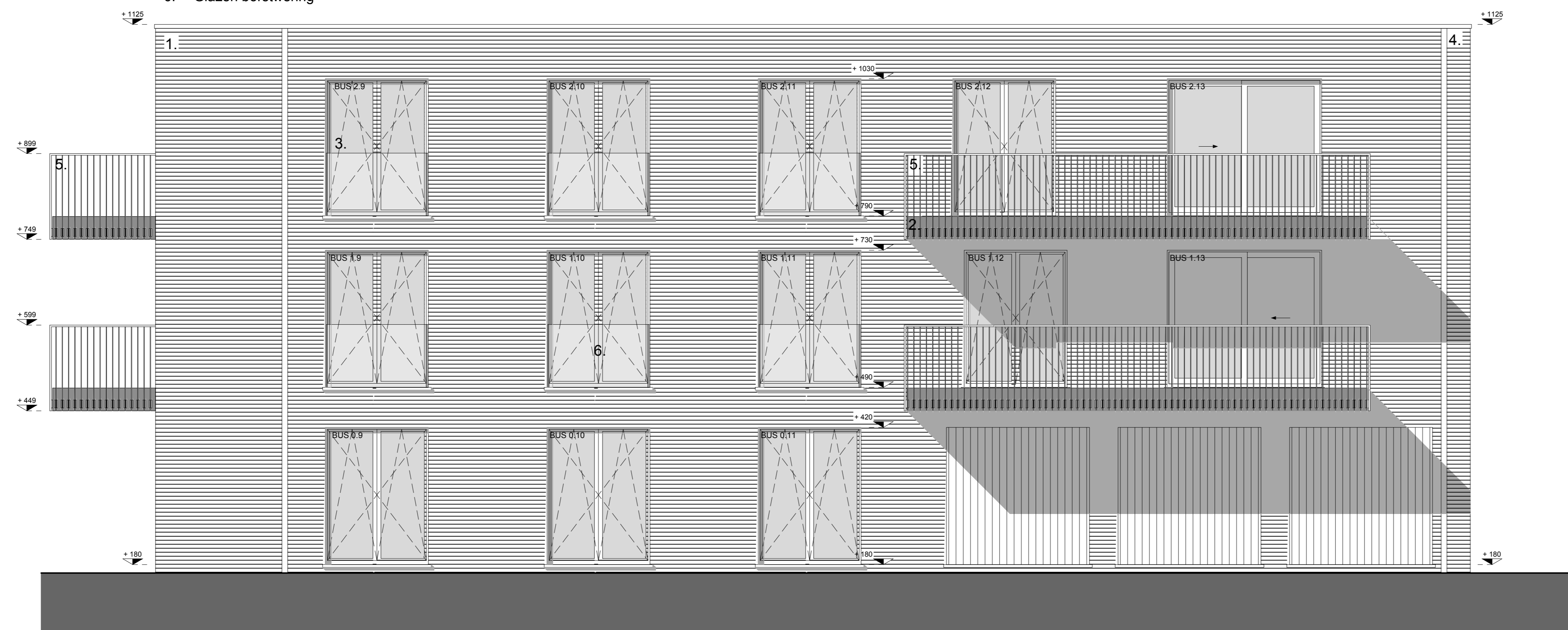
Oostgevel - Volume II 0 0,5 2,5m
