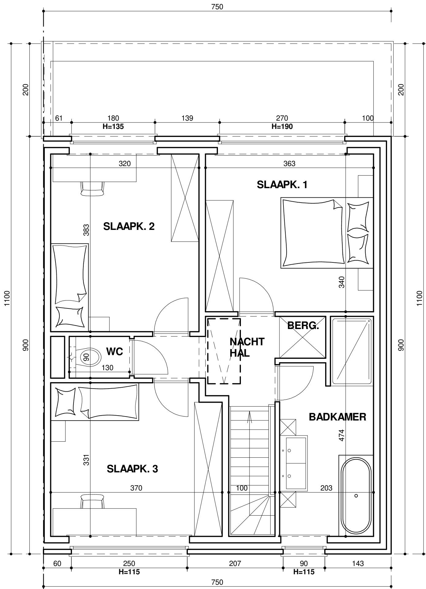
VERDIEPINGSPLAN
